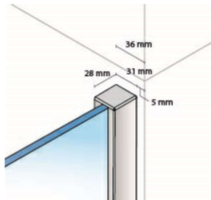
Detalle bisagra
