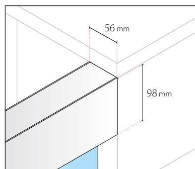
Detalle pinza
