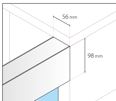
Detalle pinza
